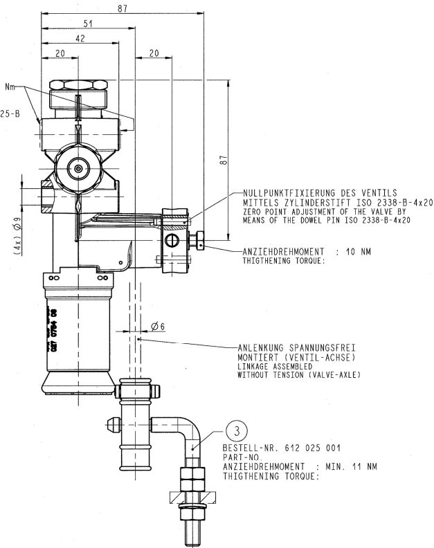
AUSFUEHRUNG: "b" CONSTRUCTION
