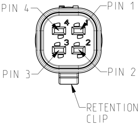
DETAIL D 2:1
